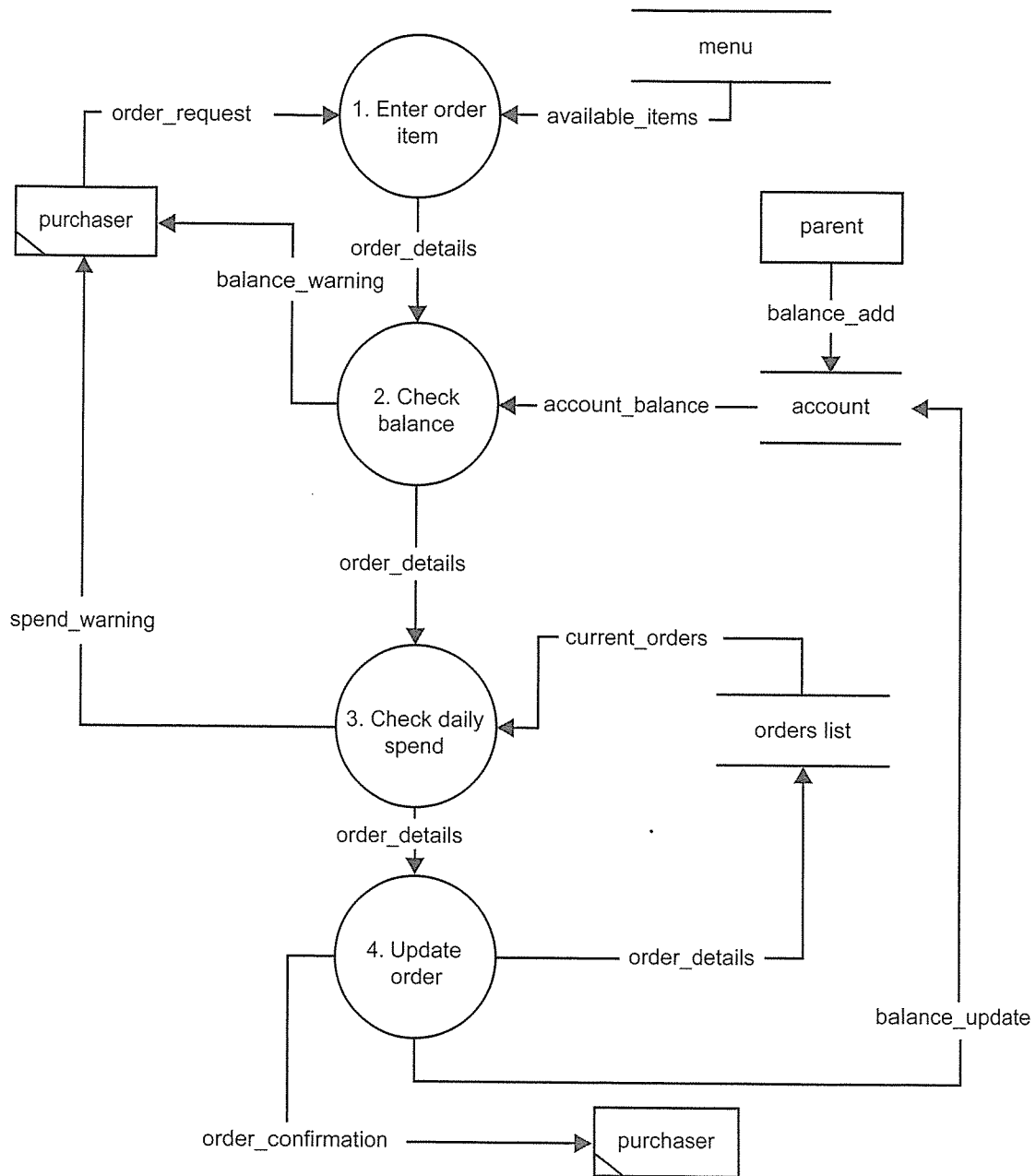
Level 0 DFD – IszCool Canteen module
